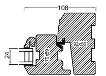
JAMB
