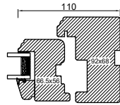
JAMB
